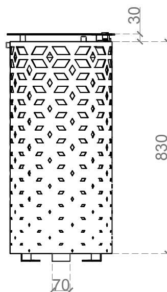
VISTA LATERAL
