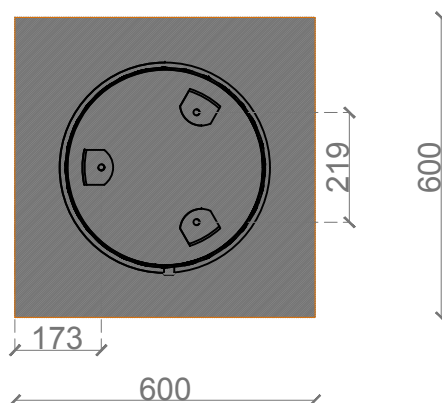
PLANTA - ESQUEMA DE MACIÇOS
