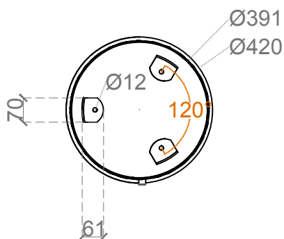
VISTA INFERIOR
