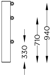
ALÇADO LATERAL SIDE VIEW
