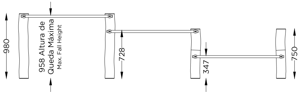
ALÇADO FRONTAL FRONT VIEW
