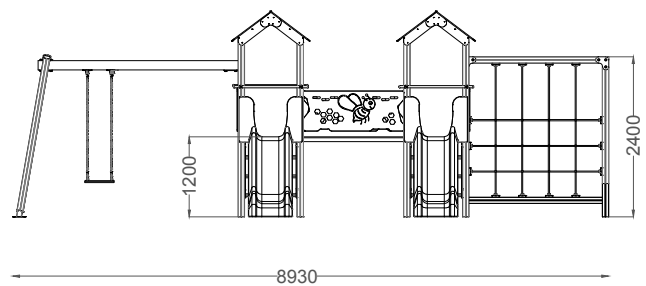
ALÇADO FRONTAL FRONT VIEW
