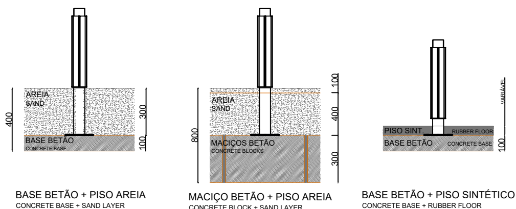
PLANTA . ESQUEMA DE FIXAÇÃO PLAN . INSTALLATION PLAN
