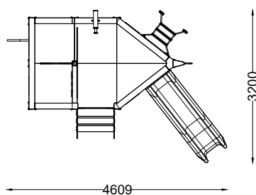
PLANTA PLAN
