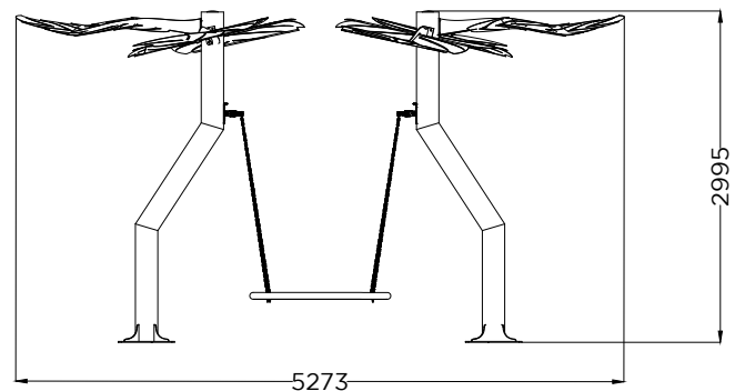
ALÇADO FRONTAL FRONT VIEW
