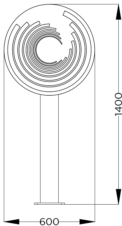
ALÇADO FRONTAL FRONT VIEW
