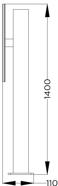
ALÇADO LATERAL SIDE VIEW
