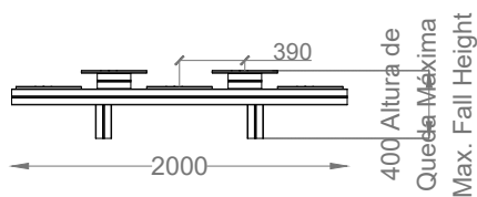
ALÇADO LATERAL SIDE VIEW
