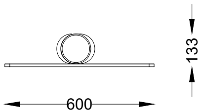
PLANTA PLAN
