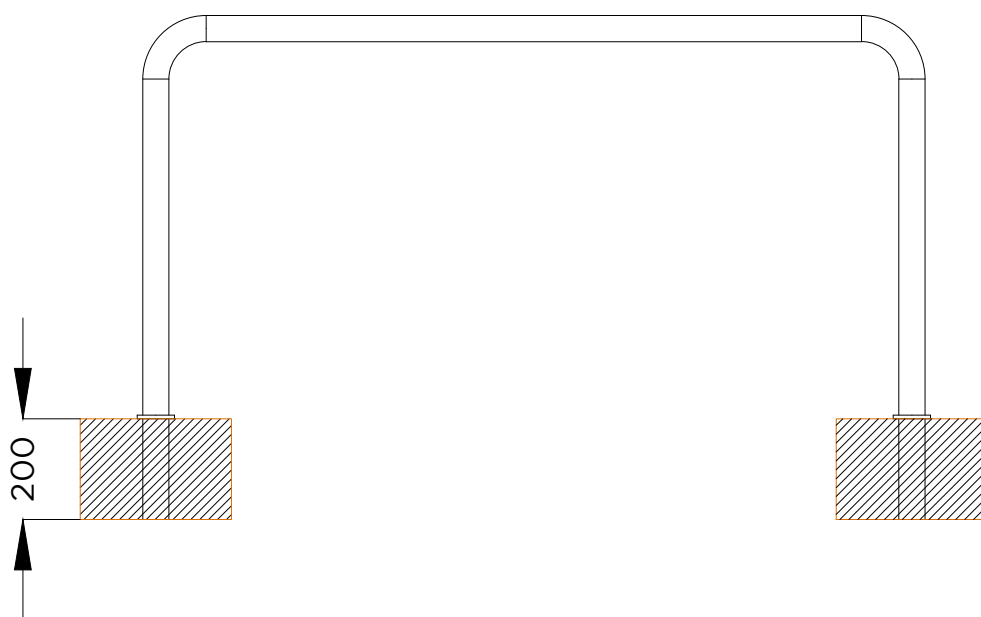
ALÇADO . ESQUEMA DE FIXAÇÃO SIDE VIEW . INSTALLATION PLAN
