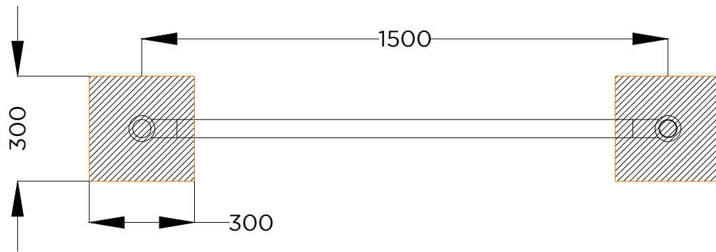
PLANTA . ESQUEMA DE FIXAÇÃO PLAN . INSTALLATION PLAN
