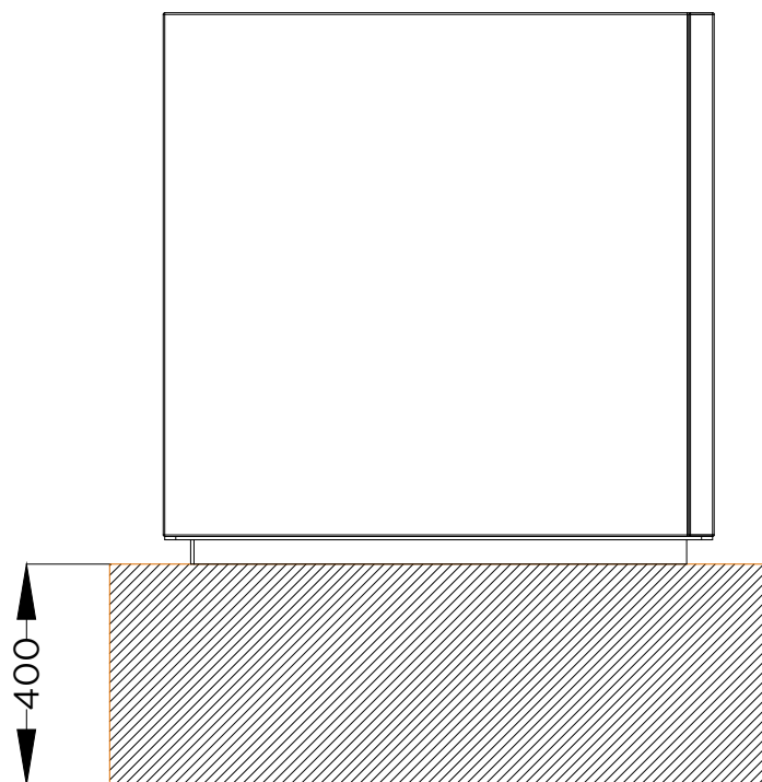
PLANTA . ESQUEMA DE FIXAÇÃO PLAN . INSTALLATION PLAN
