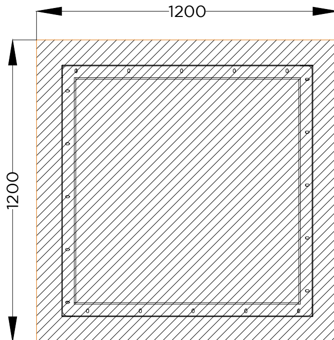
PLANTA . ESQUEMA DE FIXAÇÃO PLAN . INSTALLATION PLAN
