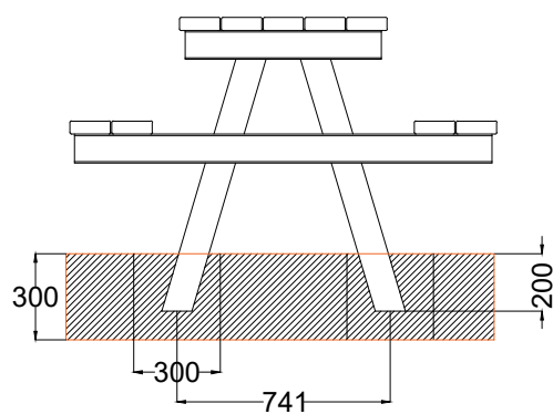
ALÇADO LATERAL . ESQUEMA DE FIXAÇÃO SIDE VIEW . INSTALLATION PLAN
