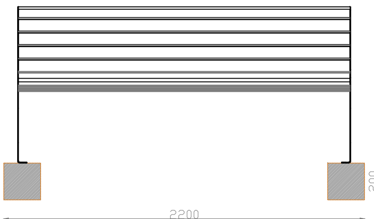
ALÇADO FRONTAL
