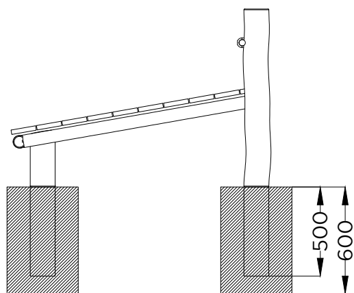
ALÇADO . ESQUEMA DE FIXAÇÃO SLIDE VIEW . INSTALLATION PLAN
