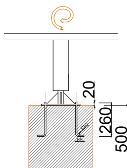
ALÇADO
