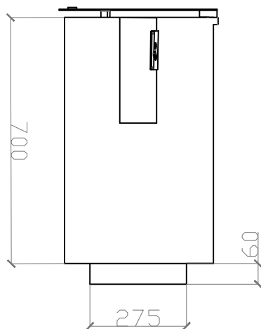
VISTA LATERAL
