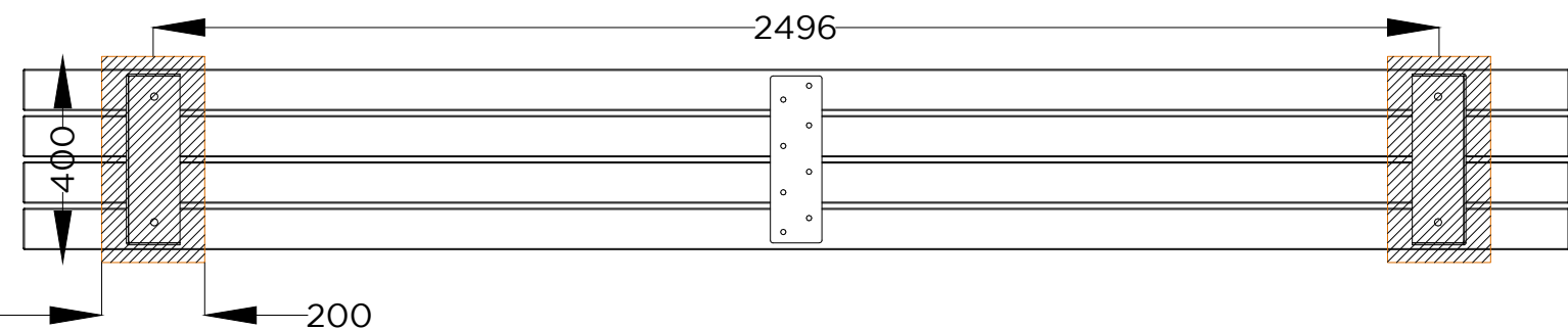
PLANTA . ESQUEMA DE FIXAÇÃO PLAN . INSTALLATION PLAN
