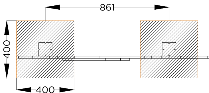
PLANTA . ESQUEMA DE FIXAÇÃO PLAN . INSTALLATION PLAN
