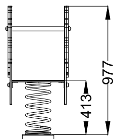
ALÇADO FRONTAL FRONT VIEW
