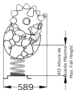
ALÇADO LATERAL SIDE VIEW
