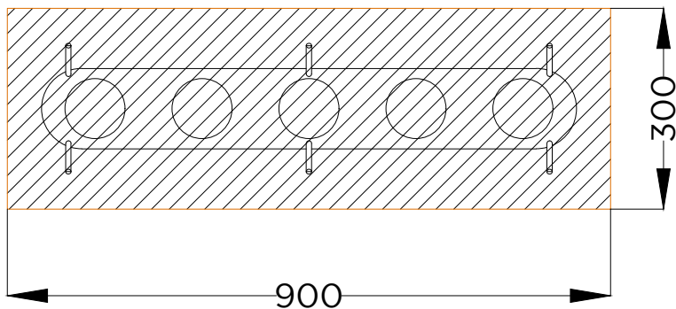
PLANTA . ESQUEMA DE FIXAÇÃO PLAN . INSTALLATION PLAN
