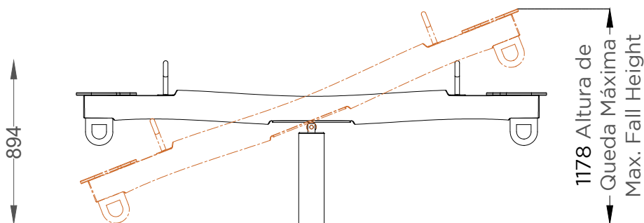
ALÇADO LATERAL SIDE VIEW
