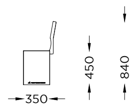
ALÇADO FRONTAL FRONT VIEW
