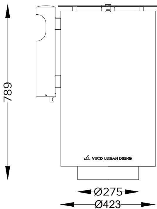
ALÇADO LATERAL SIDE VIEW
