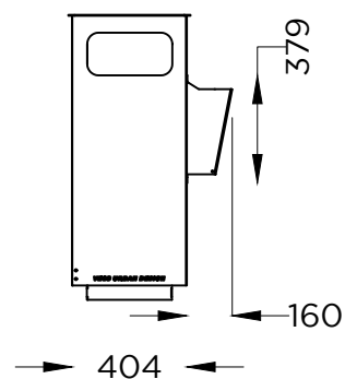
ALÇADO LATERAL SIDE VIEW
