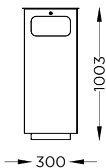
ALÇADO FRONTAL FRONT VIEW
