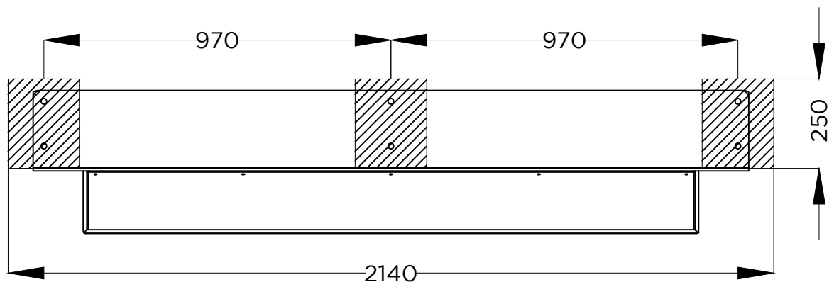
PLANTA . ESQUEMA DE FIXAÇÃO PLAN . INSTALLATION PLAN
