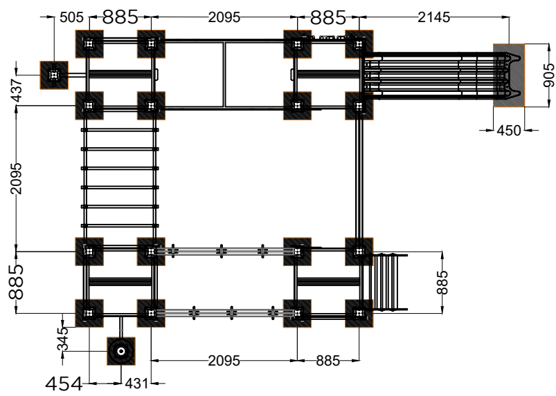
PLANTA . ESQUEMA DE FIXAÇÃO PLAN . INSTALLATION PLAN
