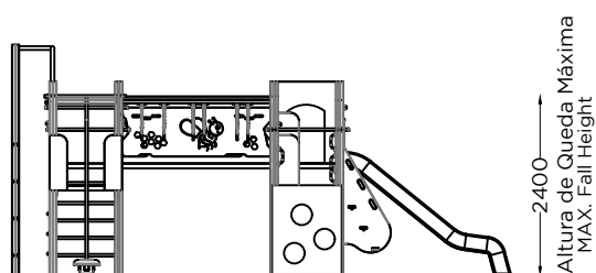
ALÇADO LATERAL SIDE VIEW
