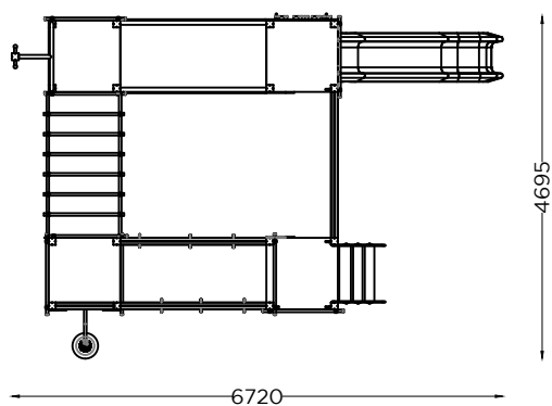
PLANTA PLAN
