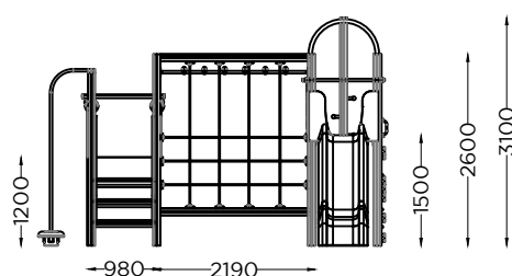
ALÇADO FRONTAL FRONT VIEW
