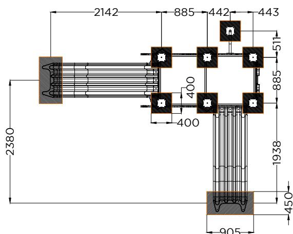
PLANTA . ESQUEMA DE FIXAÇÃO PLAN . INSTALLATION PLAN
