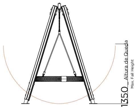
ALÇADO FRONTAL FRONT VIEW
