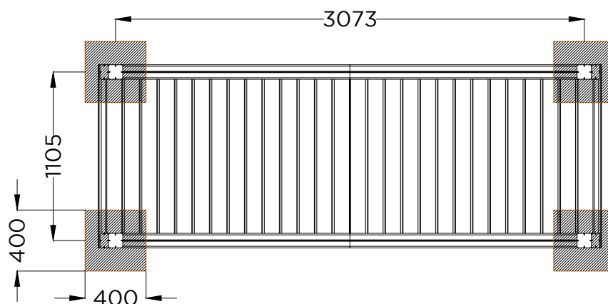
PLANTA . ESQUEMA DE FIXAÇÃO PLAN . INSTALLATION PLAN
