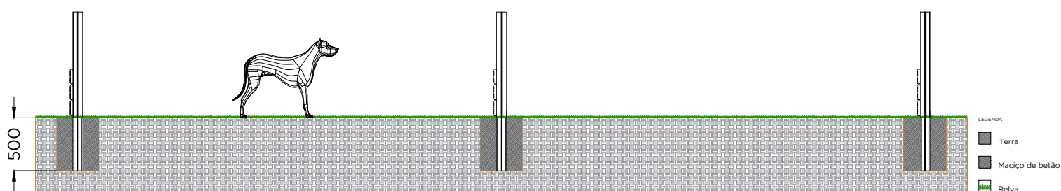
ALÇADO LATERAL . ESQUEMA DE FIXAÇÃO SIDE VIEW . INSTALLATION PLAN
