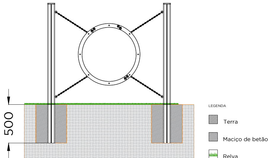
ALÇADO FRONTAL . ESQUEMA DE FIXAÇÃO FRONT VIEW . INSTALLATION PLAN
