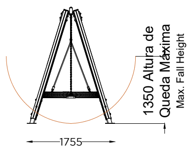
ALÇADO LATERAL SIDE VIEW
