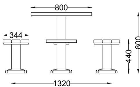
ALÇADO LATERAL SIDE VIEW
