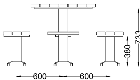
ALÇADO FRONTAL FRONT VIEW
