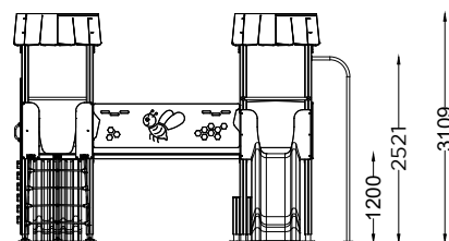
ALÇADO LATERAL SIDE VIEW
