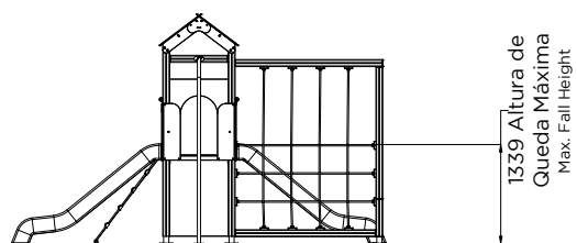
ALÇADO FRONTAL FRONT VIEW
