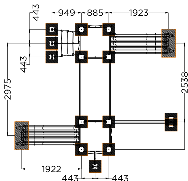
PLANTA . ESQUEMA DE FIXAÇÃO PLAN . INSTALLATION PLAN
