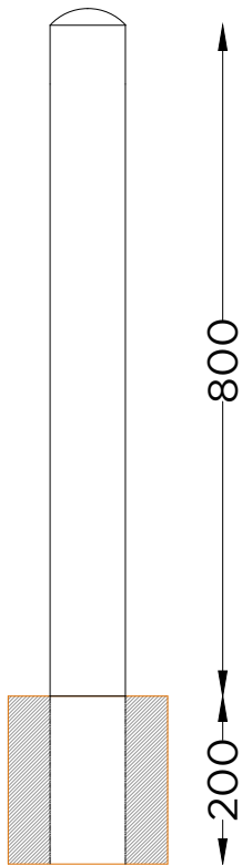
ALÇADO LATERAL SIDE VIEW
