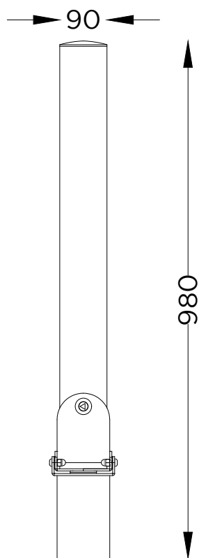
ALÇADO LATERAL SIDE VIEW
