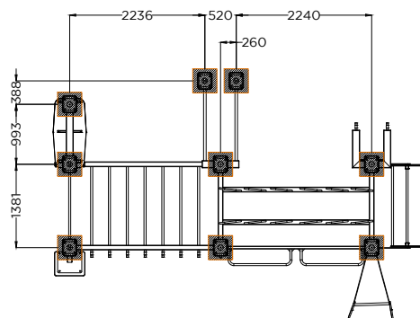
PLANTA . ESQUEMA DE FIXAÇÃO PLAN . INSTALLATION PLAN
