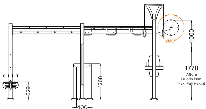
ALÇADO LATERAL SIDE VIEW
