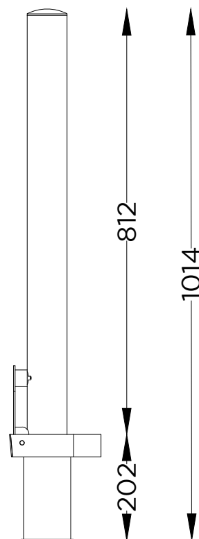
ALÇADO LATERAL SIDE VIEW
