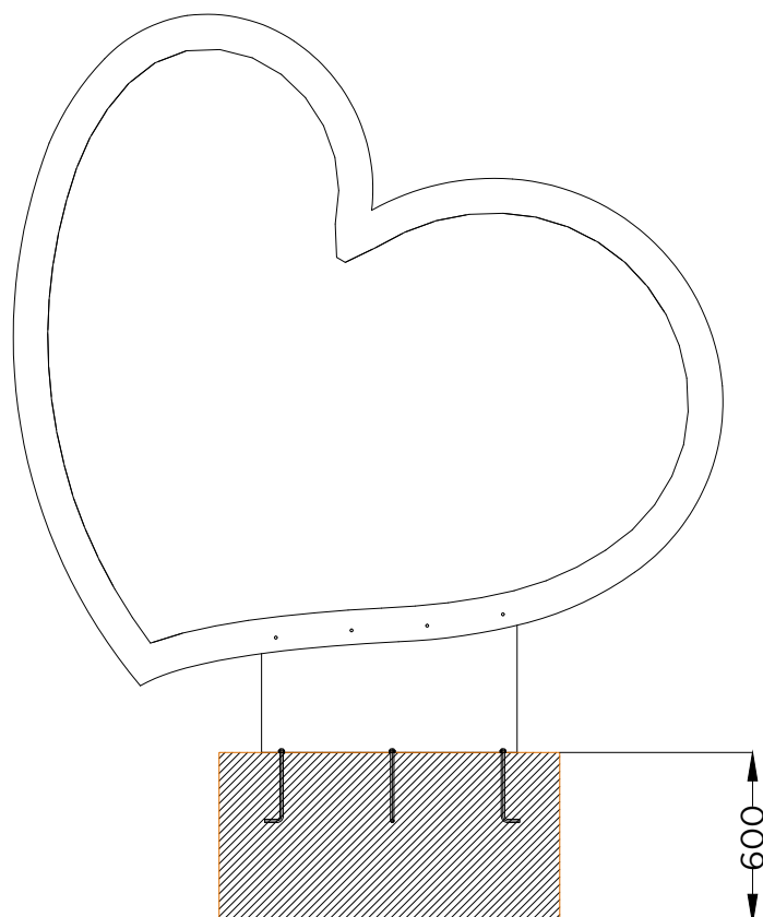
ALÇADO FRONTAL . ESQUEMA DE FIXAÇÃO FRONT VIEW . INSTALLATION PLAN
