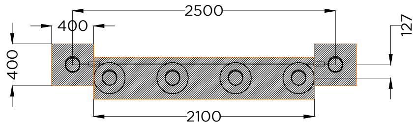
PLANTA . ESQUEMA DE FIXAÇÃO PLAN . INSTALLATION PLAN
