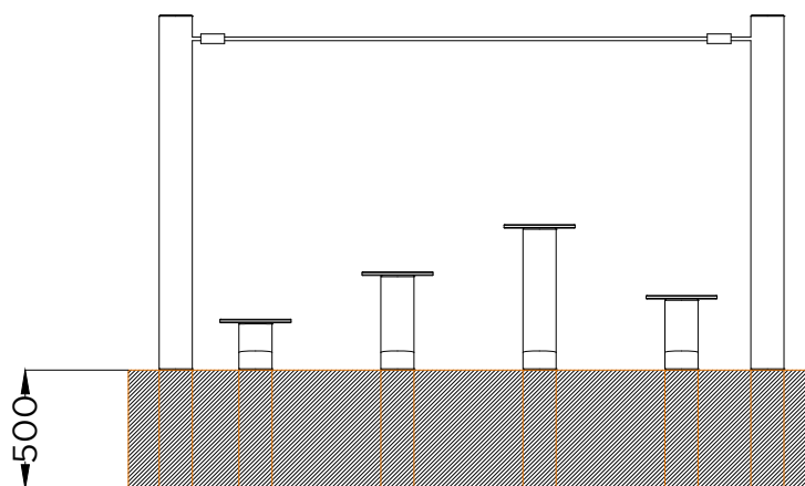
ALÇADO FRONTAL . ESQUEMA DE FIXAÇÃO SIDE VIEW . INSTALLATION PLAN
