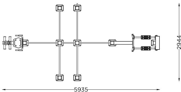
PLANTA PLAN
