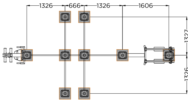
PLANTA . ESQUEMA DE FIXAÇÃO PLAN . INSTALLATION PLAN
