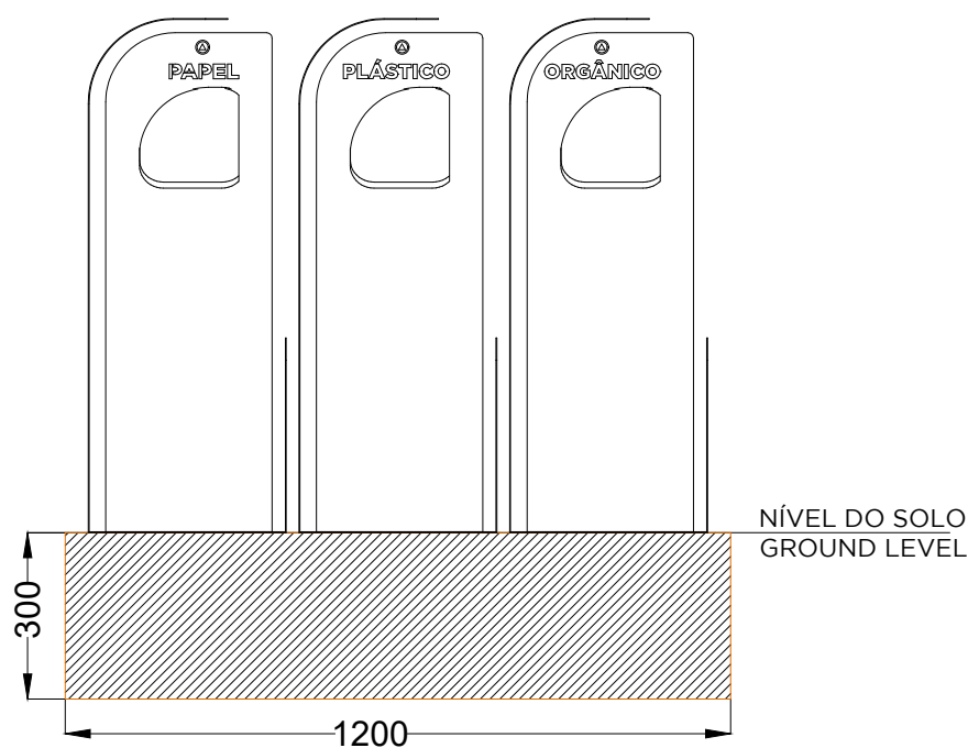
ALÇADO . ESQUEMA DE FIXAÇÃO SLIDE VIEW . INSTALLATION PLAN
