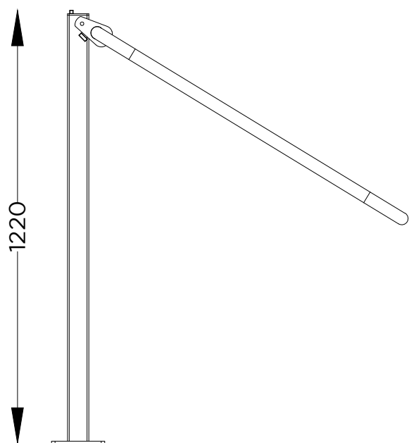
ALÇADO LATERAL SIDE VIEW
