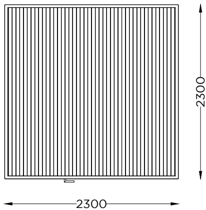
PLANTA PLAN
