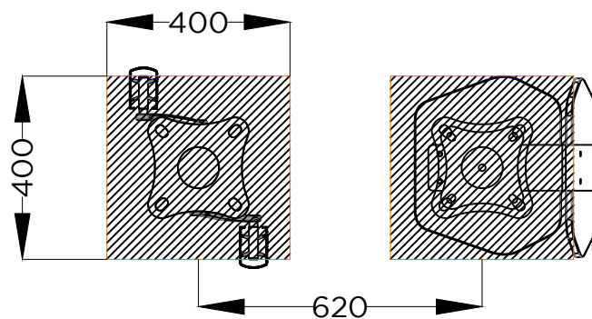
PLANTA . ESQUEMA DE FIXAÇÃO PLAN . INSTALLATION PLAN
