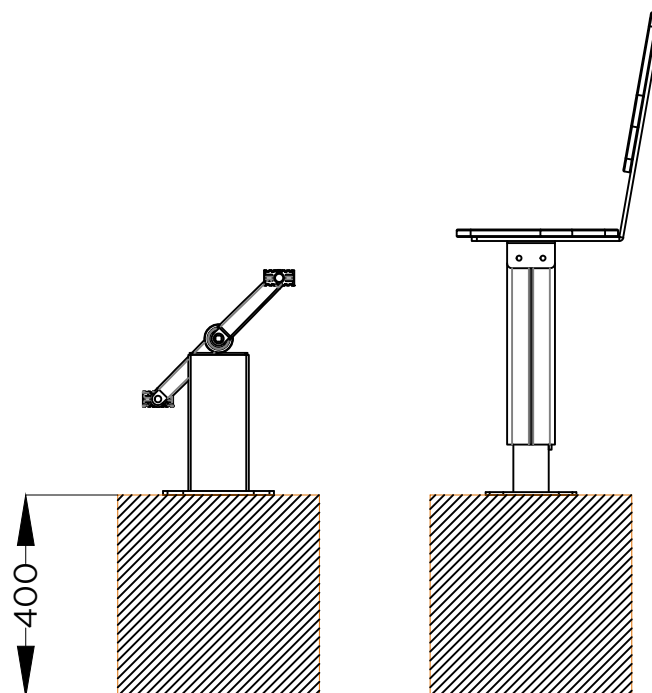
ALÇADO LATERAL . ESQUEMA DE FIXAÇÃO SIDE VIEW . INSTALLATION PLAN
