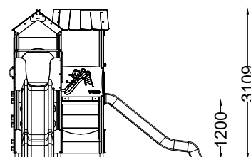
ALÇADO FRONTAL FRONT VIEW
