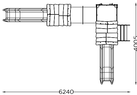
PLANTA PLAN
