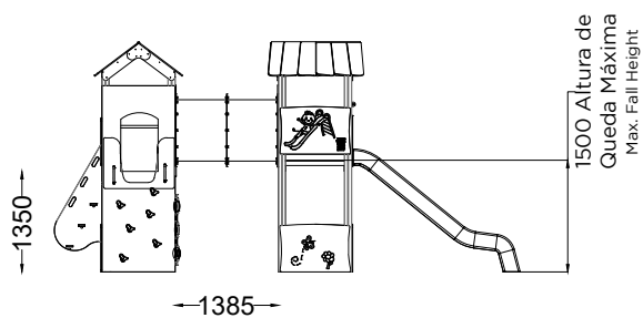
ALÇADO LATERAL SIDE VIEW
