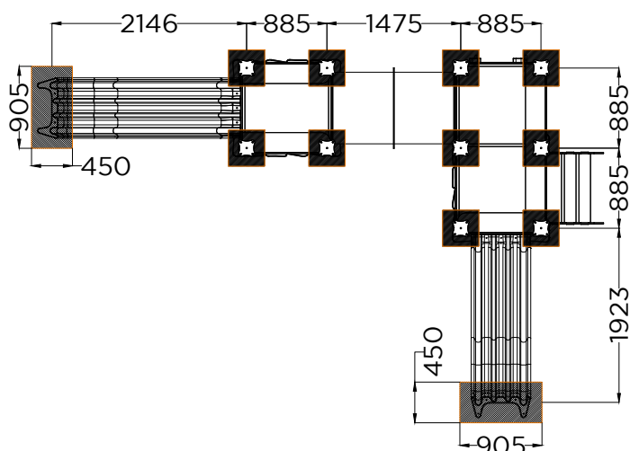
PLANTA . ESQUEMA DE FIXAÇÃO PLAN . INSTALLATION PLAN
