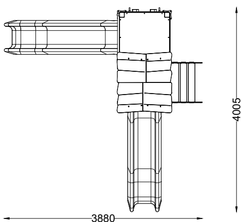
PLANTA PLAN
