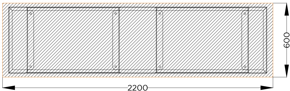
PLANTA . ESQUEMA DE FIXAÇÃO PLAN . INSTALLATION PLAN
