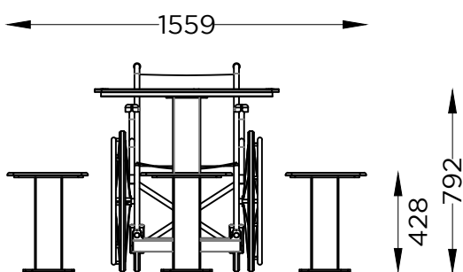
ALÇADO FRONTAL FRONT VIEW
