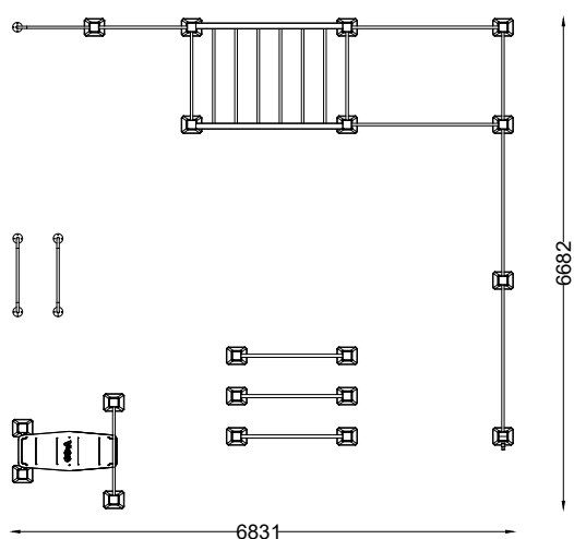
PLANTA PLAN
